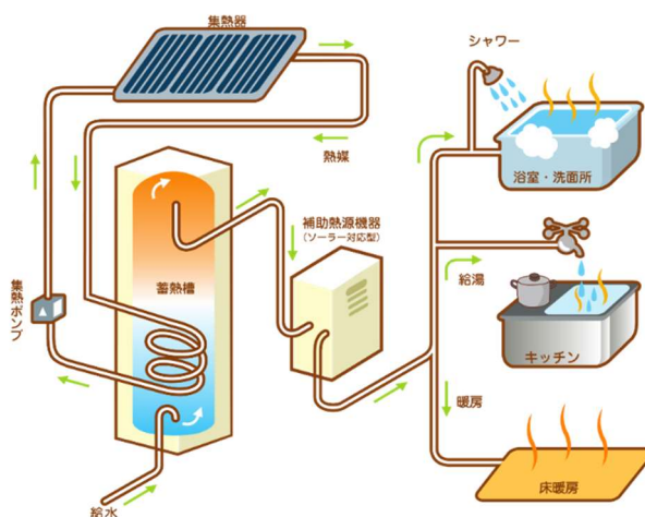
図 5.1-16 液体式ソーラーシステムの概要 出典：ソーラーシステム振興協会 HP
