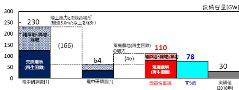
図 5.1-32 2050 年導入シナリオ【地上設置 PV 発電】
