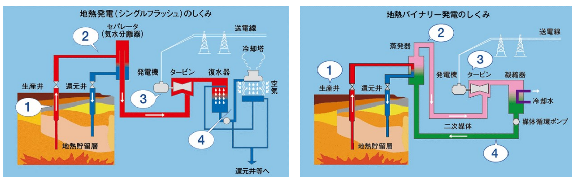
図 5.1-15 地熱発電の仕組み（左：フラッシュ発電、右：バイナリー発電） 出典：日本地熱協会 HP
